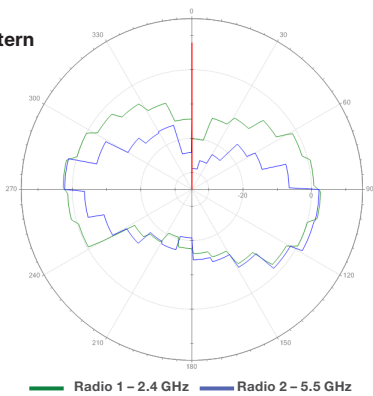
H-Plane Pattern
